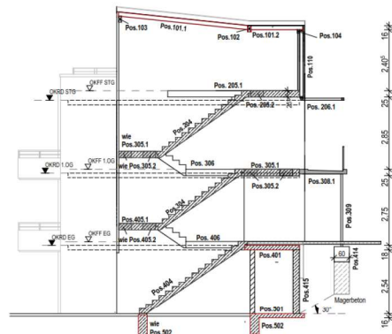
Schnitt D-D
